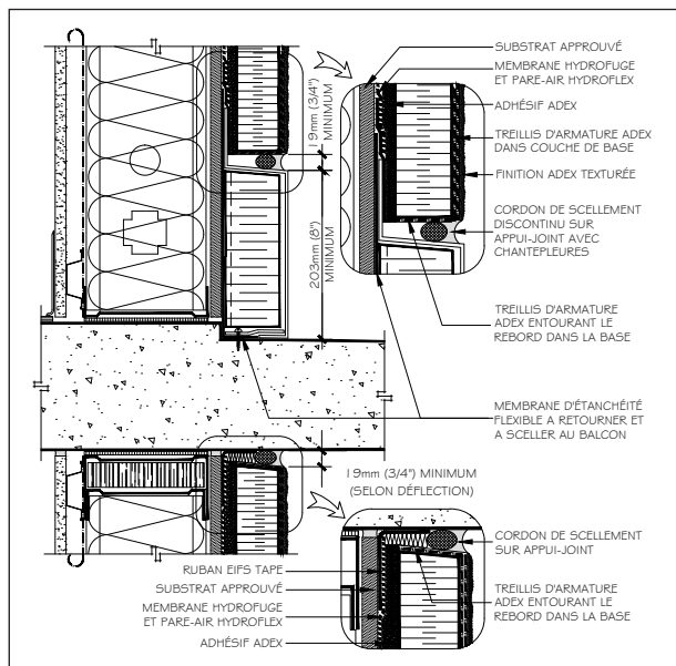
JONCTION BALCON
