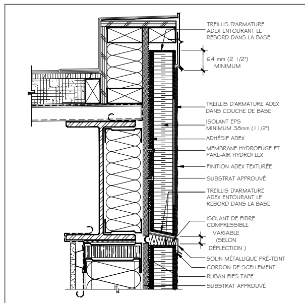
PARAPET
