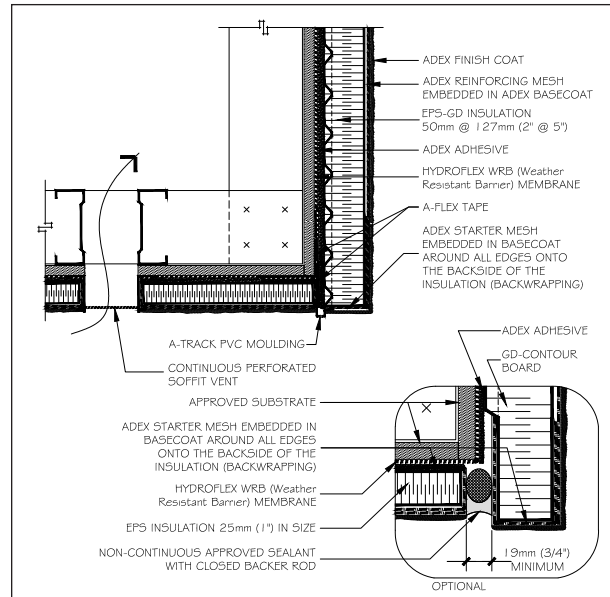
SOFFIT
