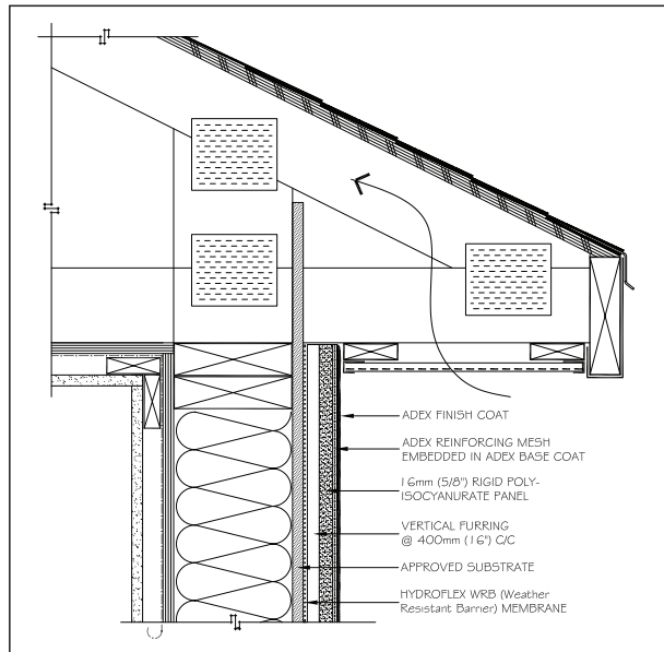
EAVE SOFFIT
